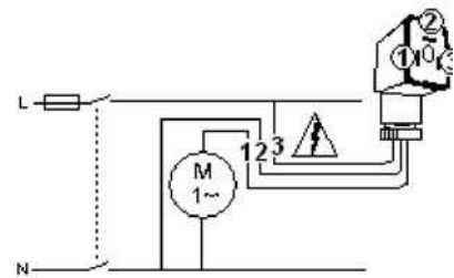
Câblage
